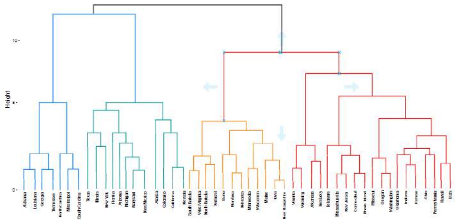
Figura 3 Exemplo de dendrograma
