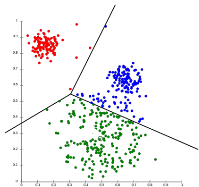
Figura 2 Exemplo de representação de dados de clusters não hierárquicos
