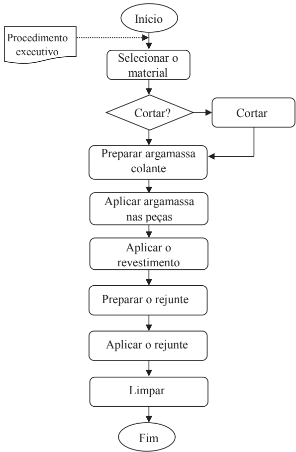
Figura 3.4 Fluxograma de processo de assentamento de revestimento cerâmico
