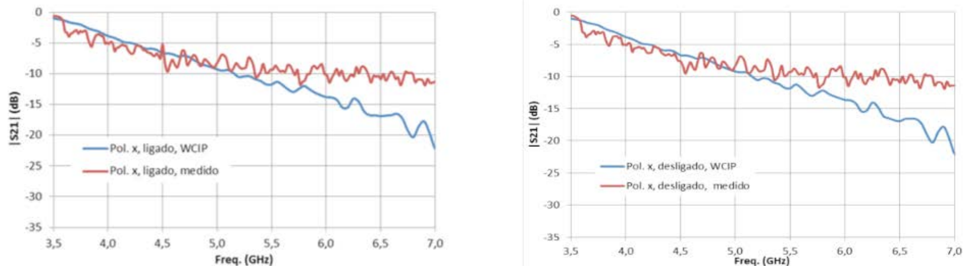
Figura 4 – Comparação da resposta em frequência, polarização x.
