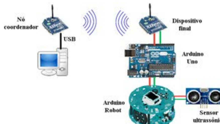
Figura 1 – Representação da plataforma experimental.
