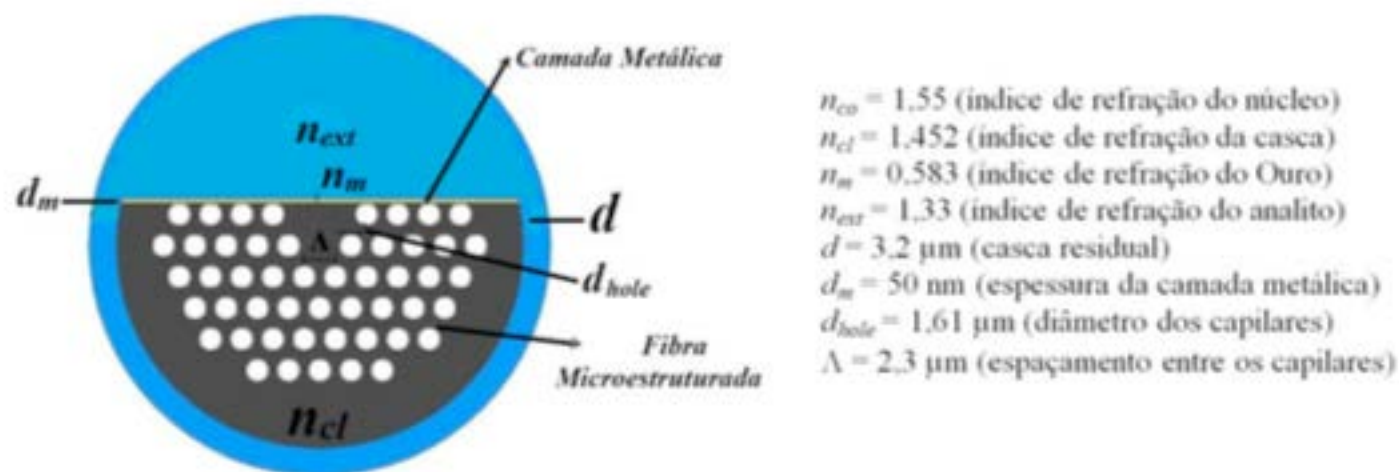
Figura 1 – Configuração adotada para a simulação do fenômeno RPS em uma fibra de cristal fotônico.
