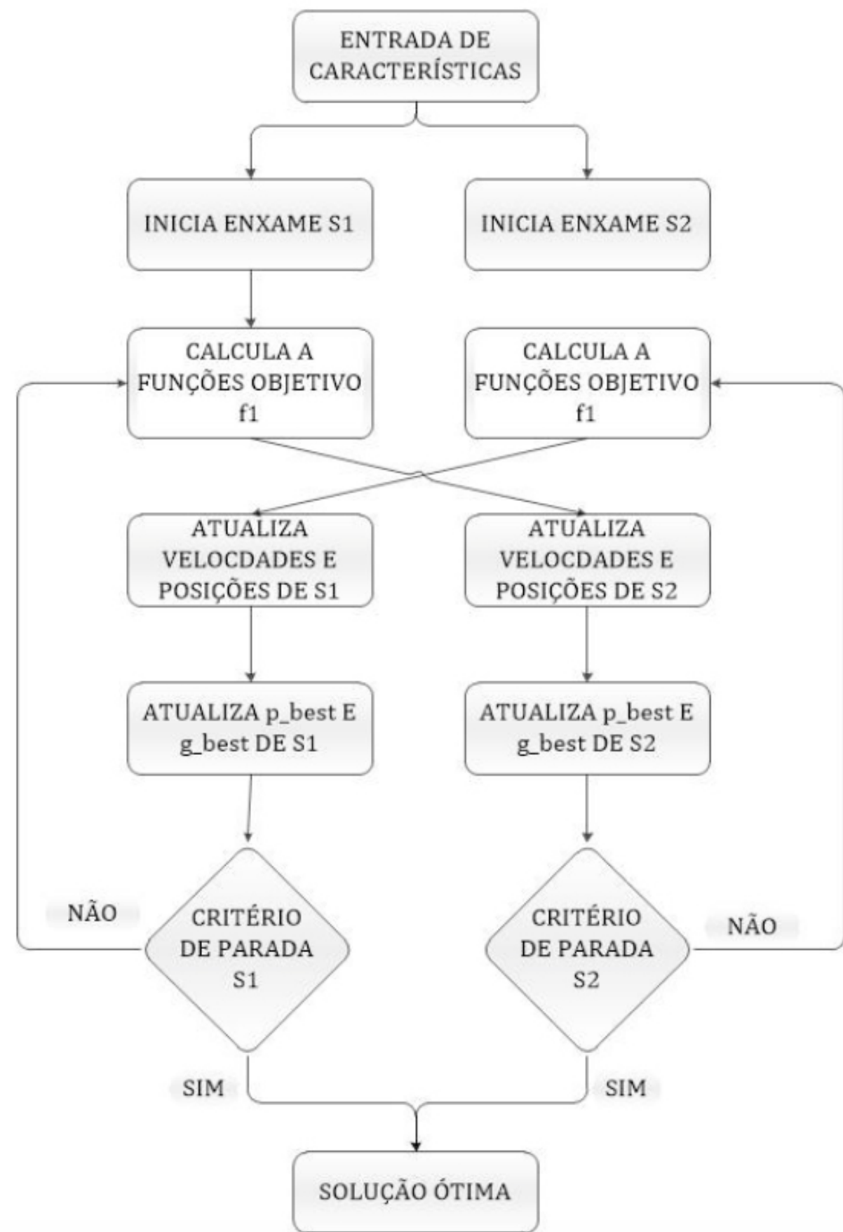
Figura 1 – Diagrama em blocos do algoritmo de otimização multiobjective VEPSO (p_best e g_best representam o melhor desempenho da partícula e o melhor desempenho do sistema, respectivamente).
