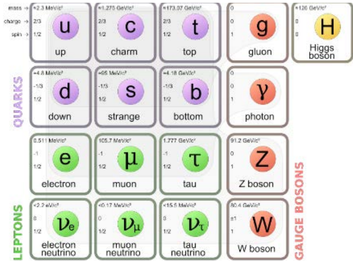
Figura 1: Tabela Periódica da Física das Partículas Elementares.
