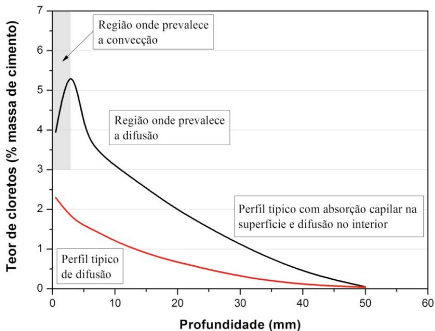
Figura 22 – Exemplo da configuração típica de perfis de cloretos onde há apenas difusão e onde prevalece a absorção capilar na superfície e a difusão no interior
