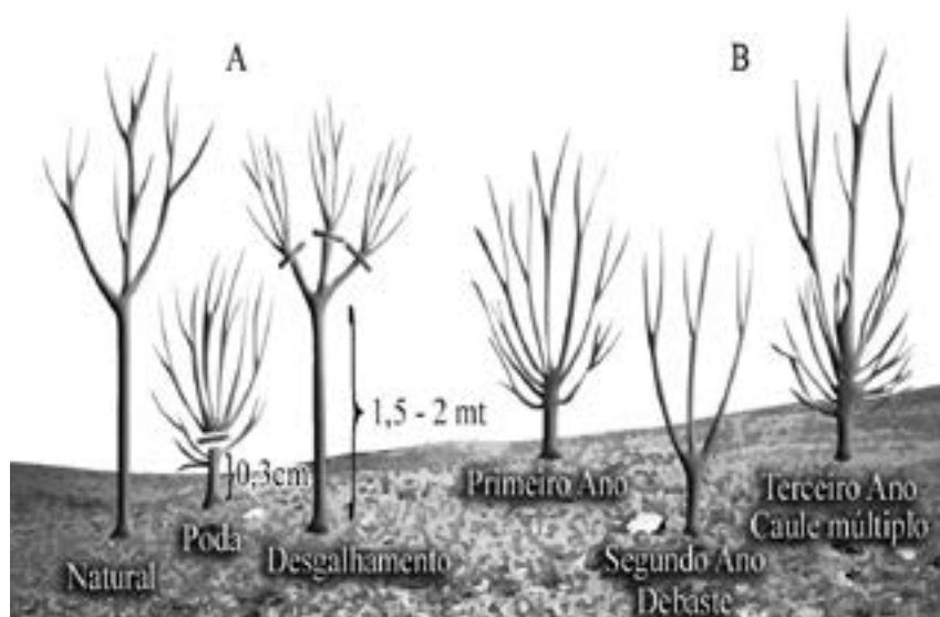
Figura 5 - Desenho esquemático das árvores com a Técnica de manejo da rebrota com altura da poda e do desganhamento (A) e evolução ao longo do tempo (B).
