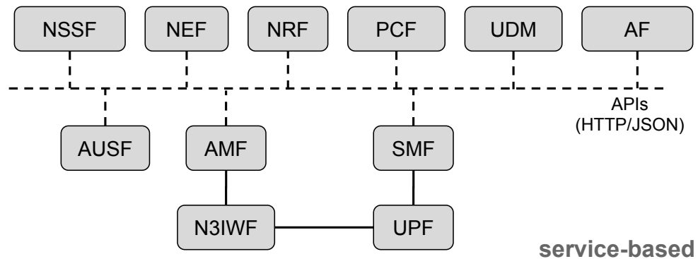
Figura 1.2 – Núcleo 5G.
