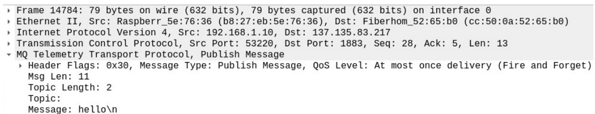
Figura 3.10 – Tela de recebimento da mensagem - Wireshark [Elaborada pelos autores].
