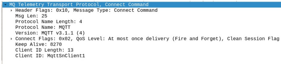
Figura 3.9 – Pacote de solicitação de conexão do ESP32 - Cliente 1 [Elaborada pelos autores].
