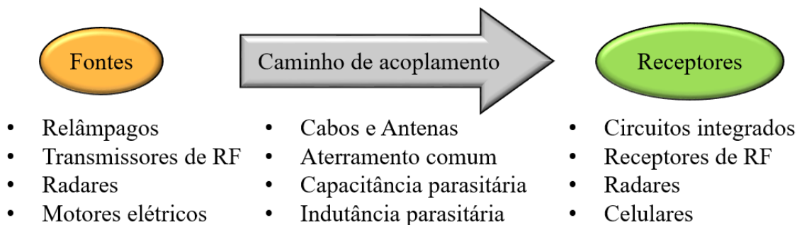
Figura 4.1 – Elementos de um problema de EMC.
