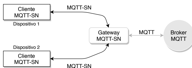
Figura 3.2 – Arquitetura.
