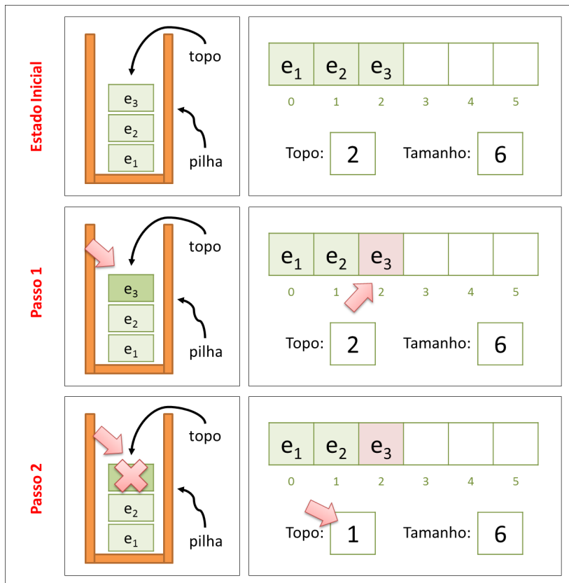
Figura 5.4 – Pilha Estática - Operação Pop
