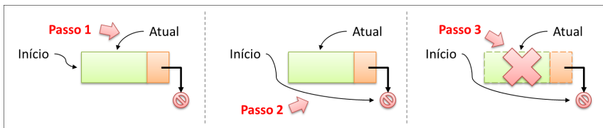
Figura 4.16 – Lista Simplesmente Encadeada - Remover do Início com um único nó
