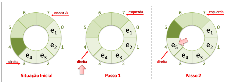
Figura 7.4 – Deque Estático - Inserir à Direita
