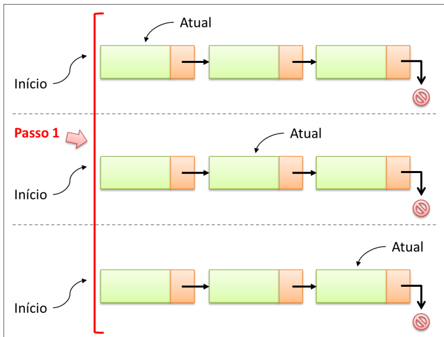
Figura 4.13 – Lista Simplesmente Encadeada - Inserir no Final, localizando o último nó
