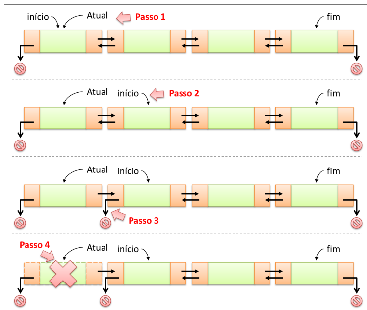
Figura 4.28 – Lista Duplamente Encadeada - Remover do Início
