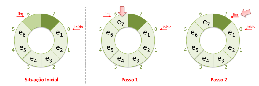
Figura 6.7 – Fila Estática Circular - Inserindo elemento
