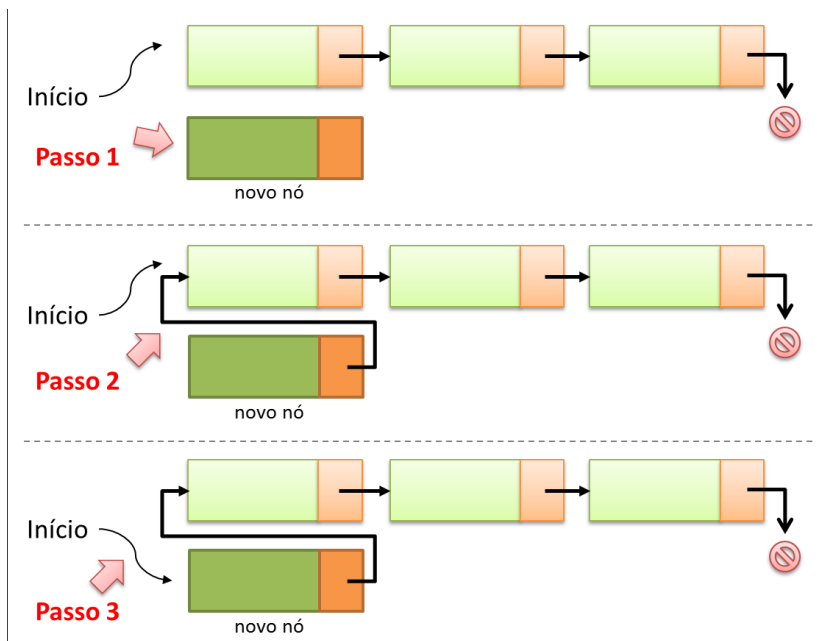
Figura 4.11 – Lista Encadeada Simples - Inserir no Início
