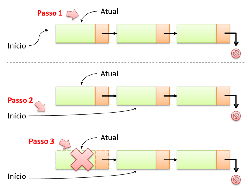
Figura 4.15 – Lista Encadeada - Remover do Início
