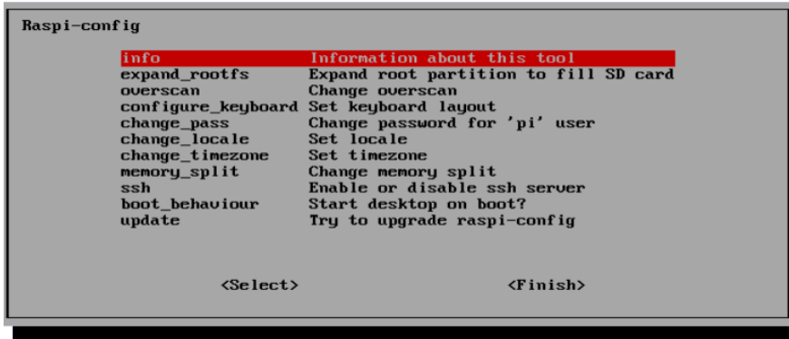
Figura 12 – Raspi-config
