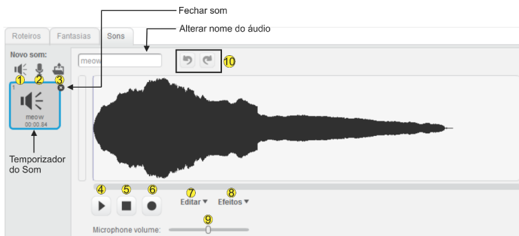
Figura 29 – Aba Sons
