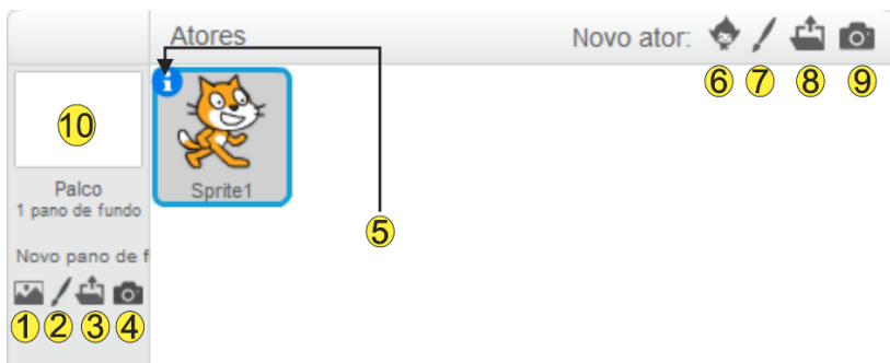
Figura 23 - Atores
