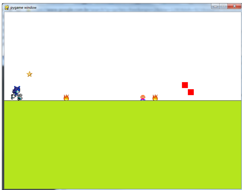
Figura 116 – Jogo Superpygame
