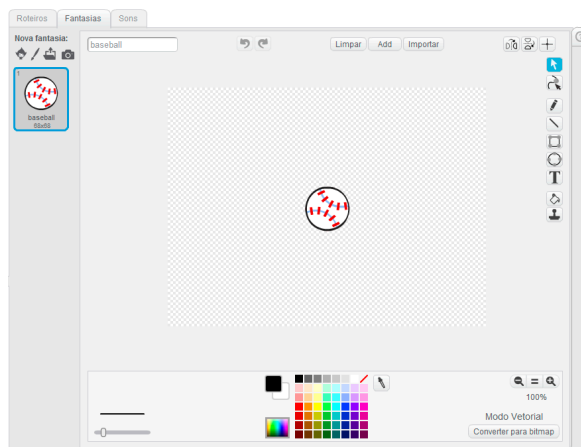
Figura 68 – Personagem Bola
