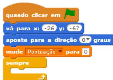
Figura 73 – Comando Sempre
