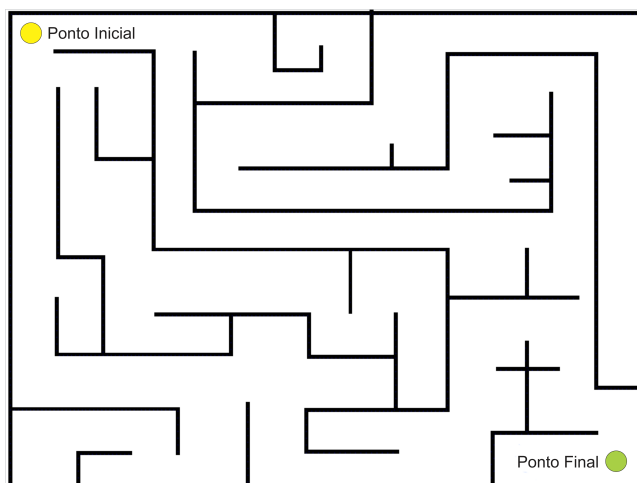
Figura 35 – Palco labirinto
