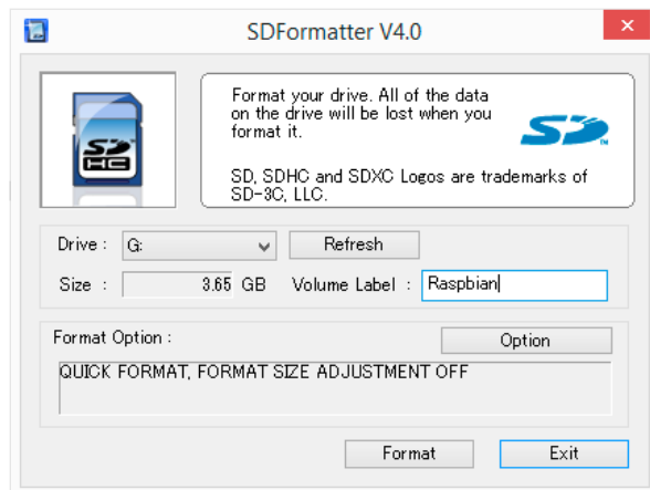
Figura 9 – Format Option
